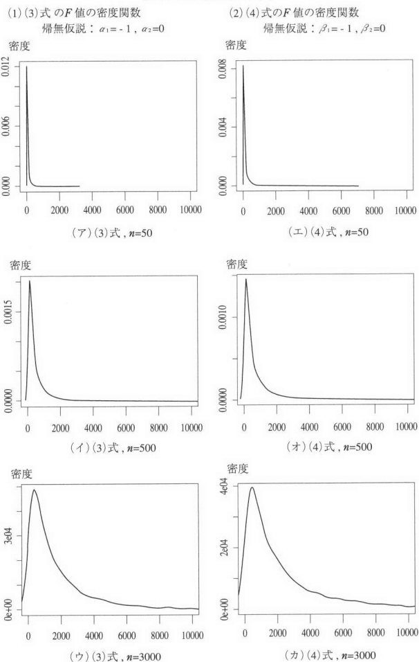
図4. (3)式, (4)式の F 値のシミュレーション結果: 繰り返し回数 10000 回
