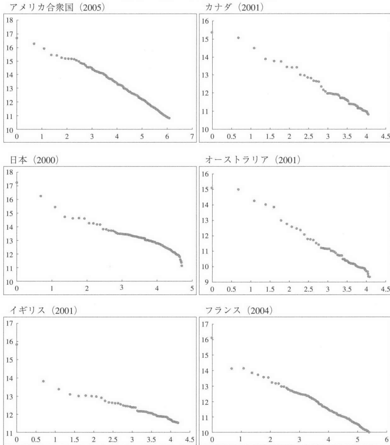
図1. 各国都市の人口規模と順位の散布図 (横軸: \log(\text{rank}) , 縦軸: \log(\text{Size}) )
