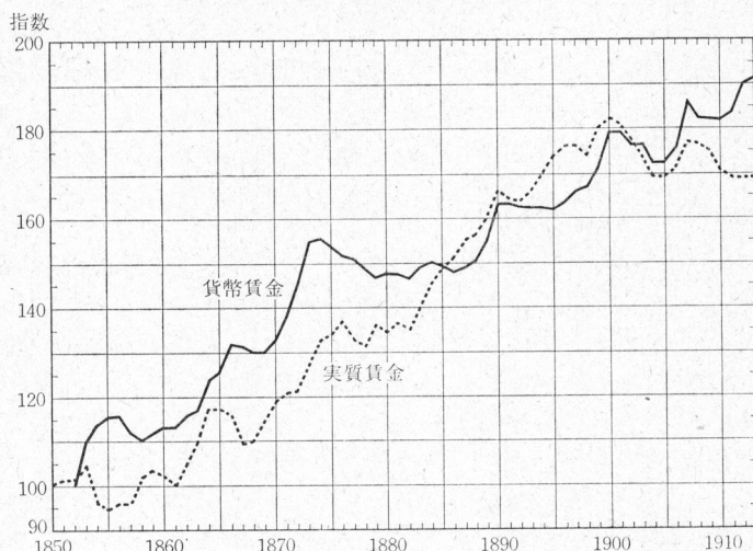
第1図 貨幣賃金指数と実質賃金指数
