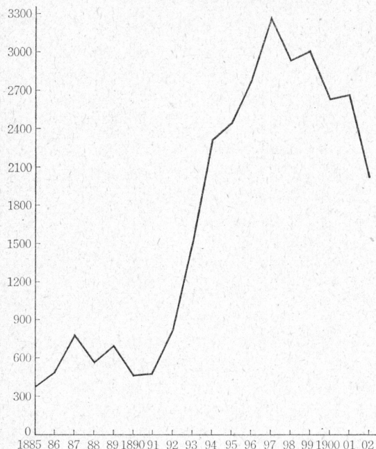
第2図 社会民主連盟のメンバー数
